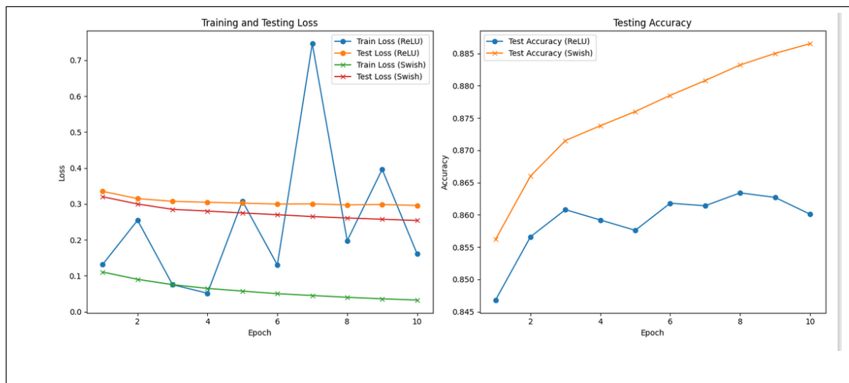
شکل ۹. مقایسه عملکرد الگوریتم یادگیری عمیق با تابع Swish و ReLU Fig. 9. Comparison of the performance of the deep learning algorithm with the swish and relu functions
