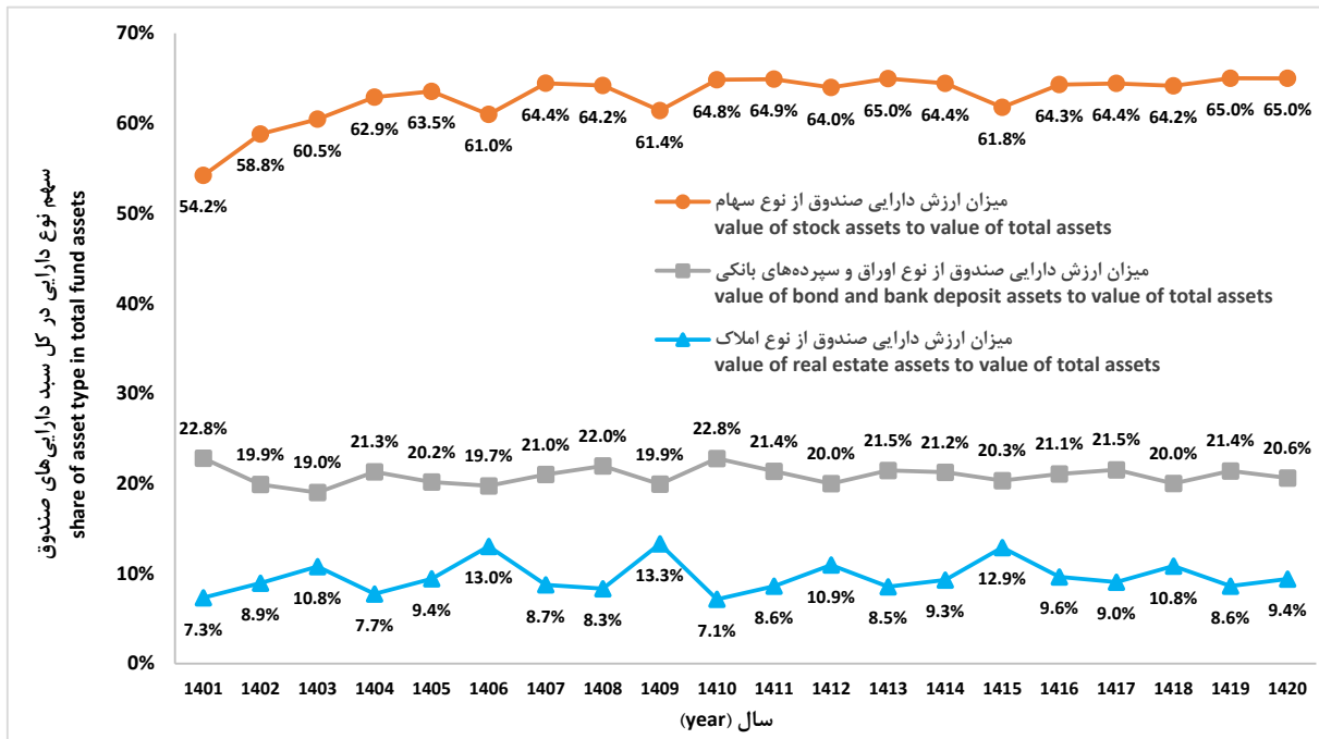
نمودار ۲: نتایج اجرای مدل برنامه‌ریزی تصادفی برای پیش‌بینی تخصیص منابع صندوق Fig. 2: Results of implementing proposed stochastic programming model for allocation of the Fund assets
